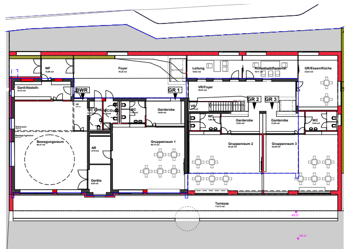
Die Raumeinteilung im Erdgeschoss
